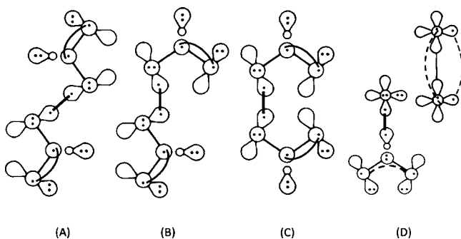
Figure 3. GVB diagrams for (A–C) O–O dimers and (D) NO + NO 3 − ionic pair.
